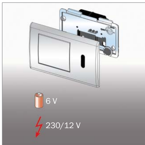
Moduł elektroniki do WC TECEplanus z czujnikiem podczerwieni. Bezdotykowe uruchamianie spłukiwania. Zasilanie odbywa się bateryjnie lub z sieci.
