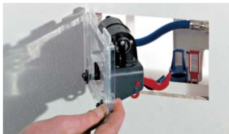
Płytką osłonową z zamontowanym siłownikiem przeznaczonym do współpracy z modułem elektroniki uruchamianej na podczerwień, jak również przyciskiem elektrycznym.
