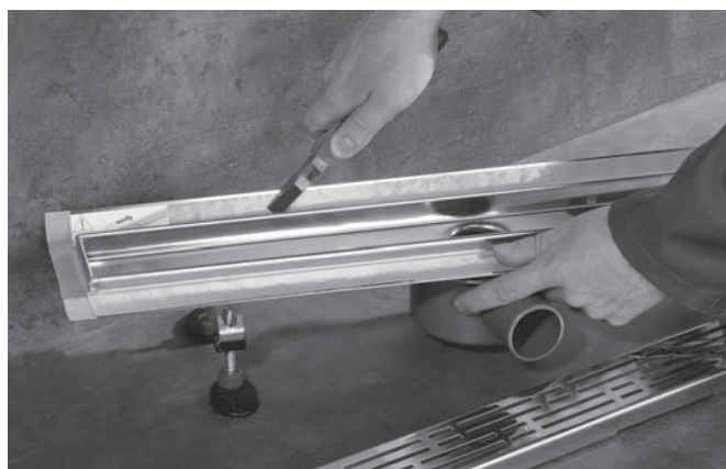
Rozkładanie kołnierza rynny prysznicowej przed zabudowaniem
