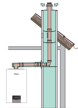
Przyłącze do przewodu spalinowego \varnothing 80 mm (w szachcie)
